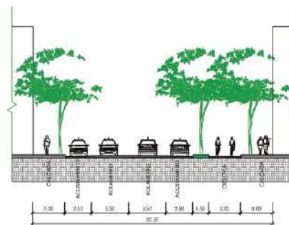
VIA COLETORA III COM CICLOVIA
