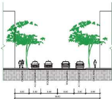
VIA COLETORA III SEM CICLOVIA
