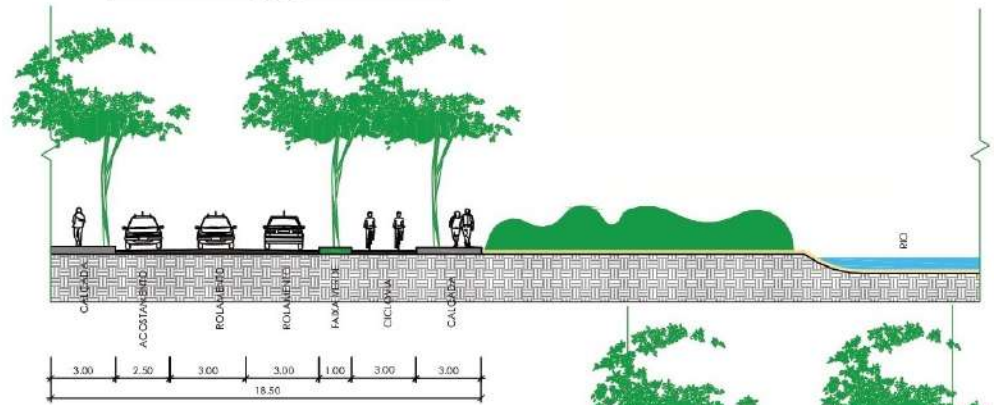
VIA DE CONTENÇÃO II
