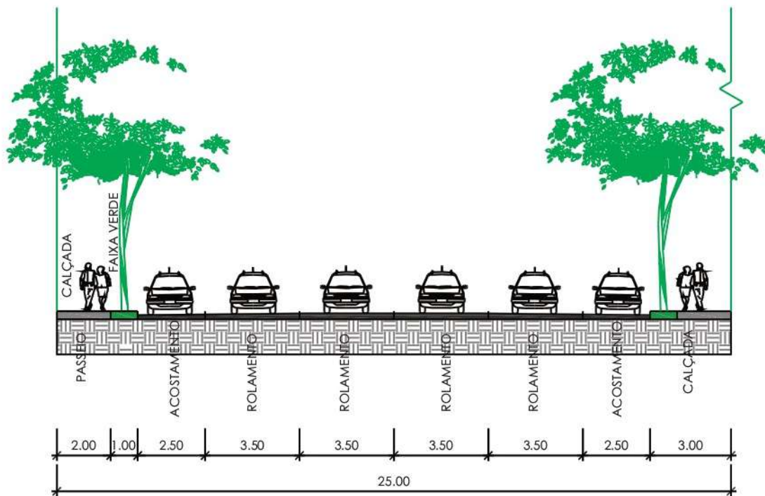
VIA COLETORA II
