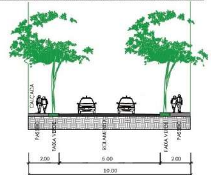
VIA INTERNA DE CONDOMÍNIO
