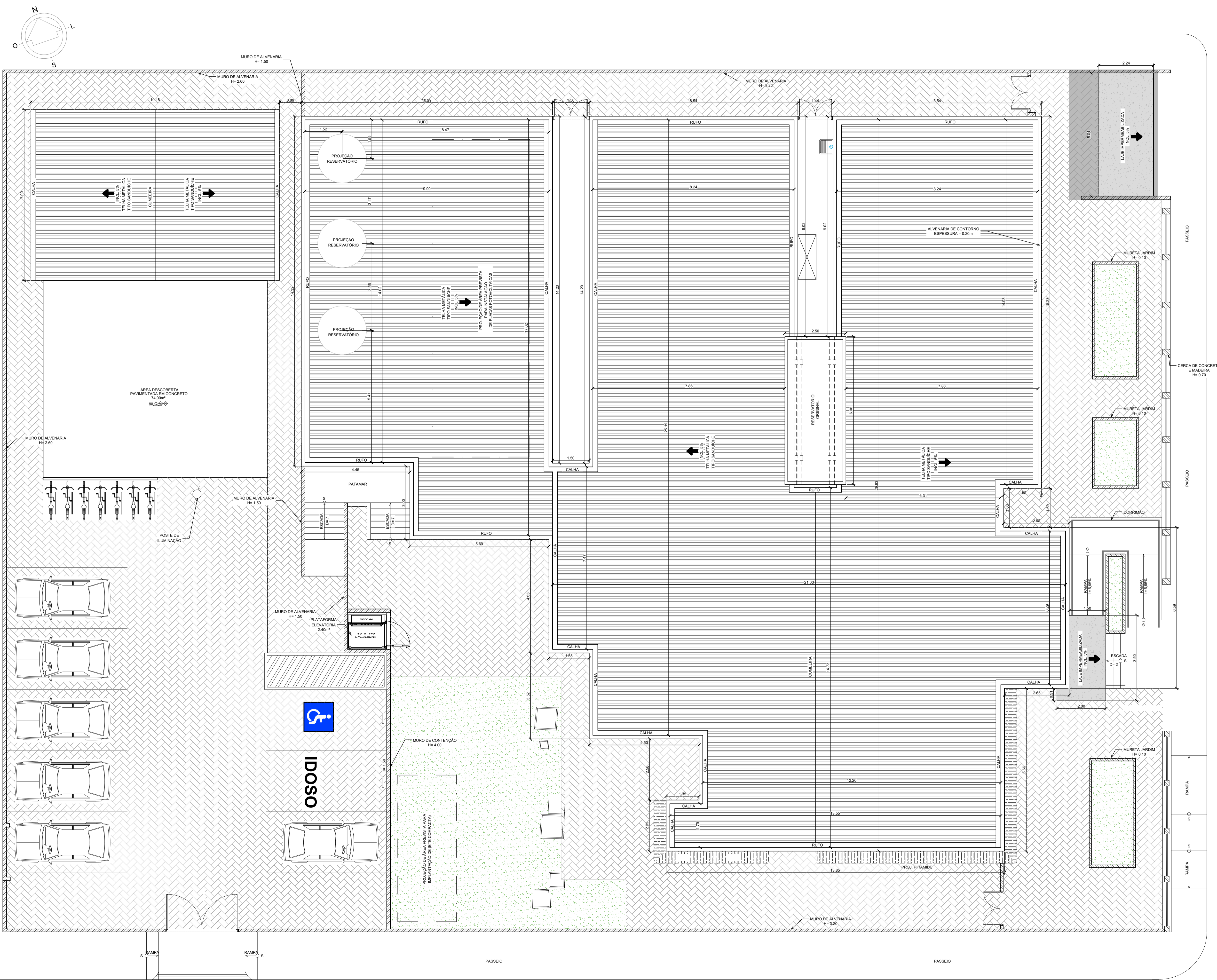
PLANTA DE IMPLANTAÇÃO COM COBERTURA
